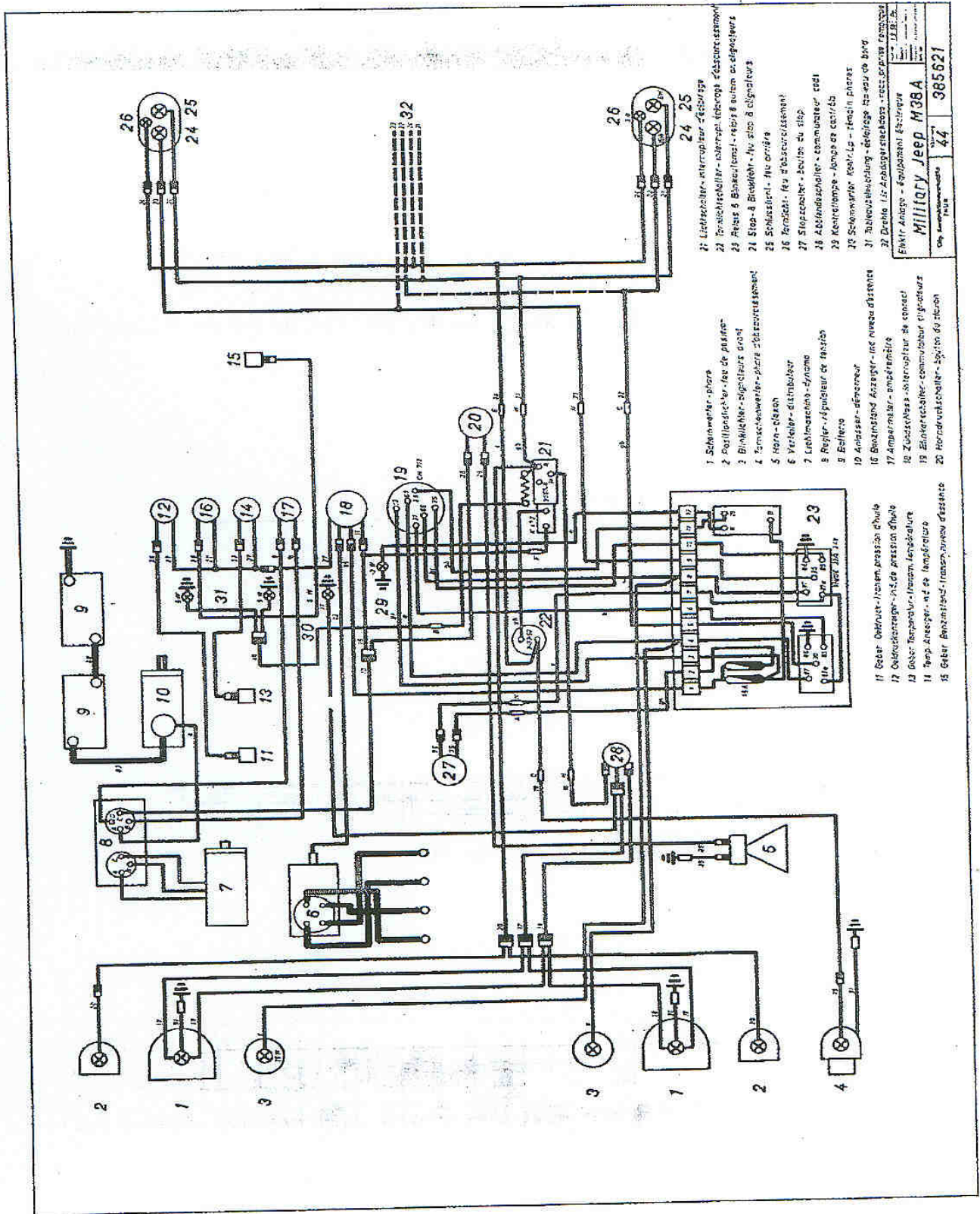
Fig. 36 Schéma des connexions avec les agrégats et les numéros indicatifs de câbles
