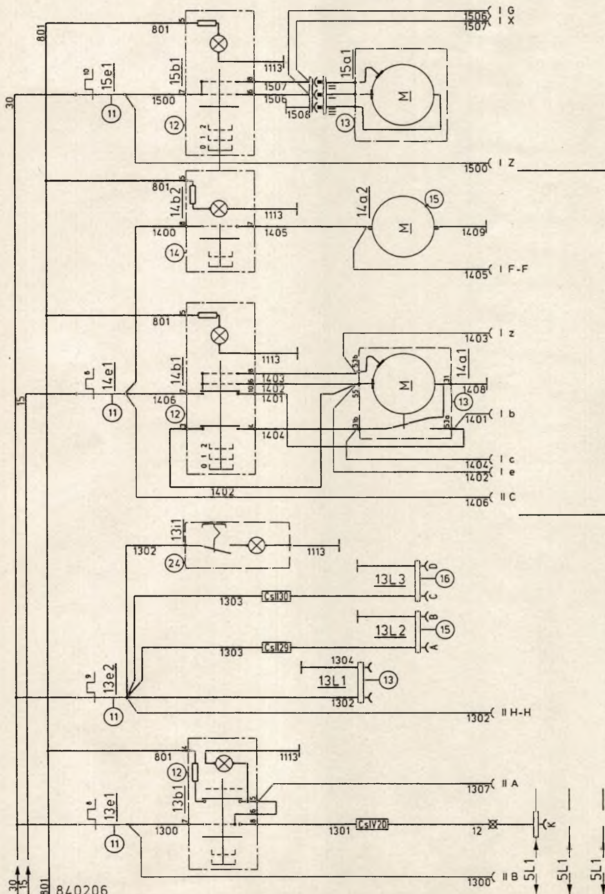
Heizgebläse Bild Nr. 1280.623
