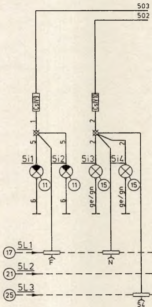
Stop-Lichter
