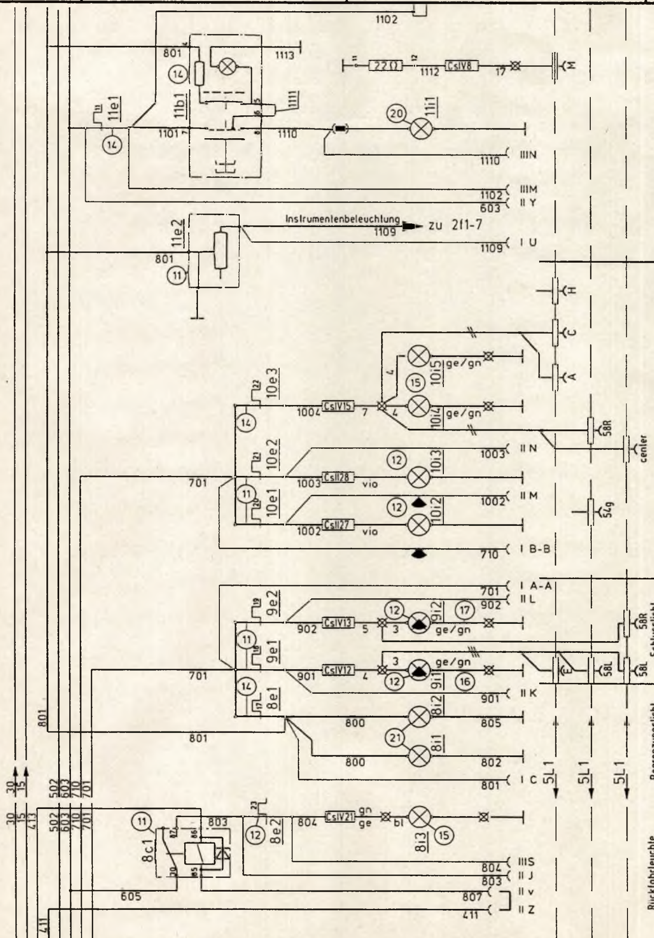
Deckenleuchte, Signalhorn
