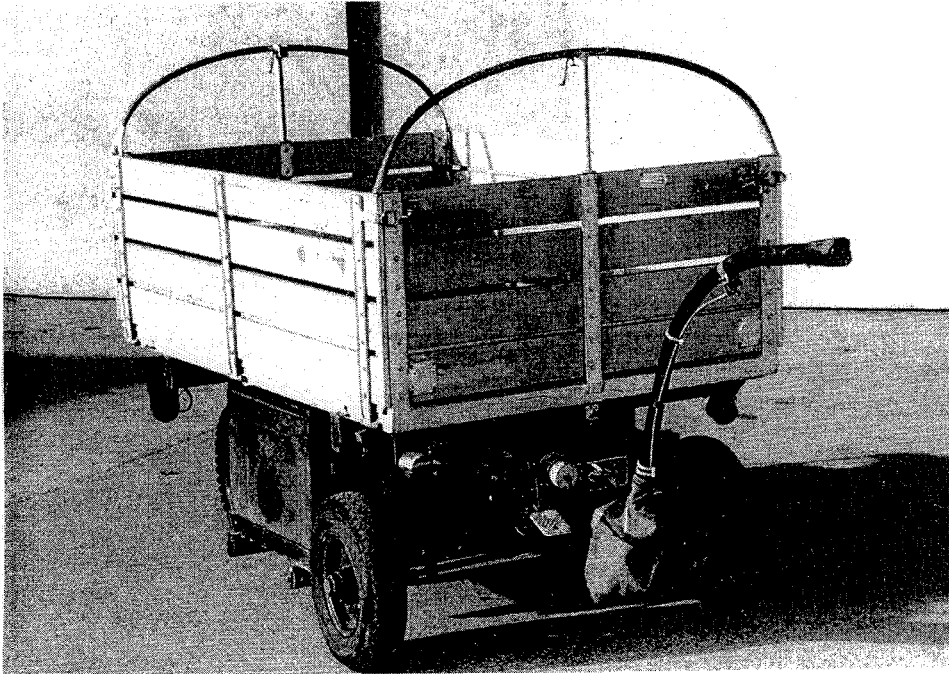
Elektro-Handfourgons I Fourgonnette électrique à timon I
